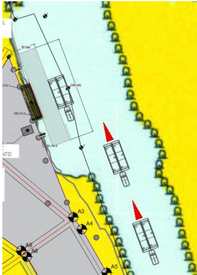
Ilustración 2. Aproximación de las barcazas al área de maniobra frente al muelle fluvial en convoy de 2 barcazas.
