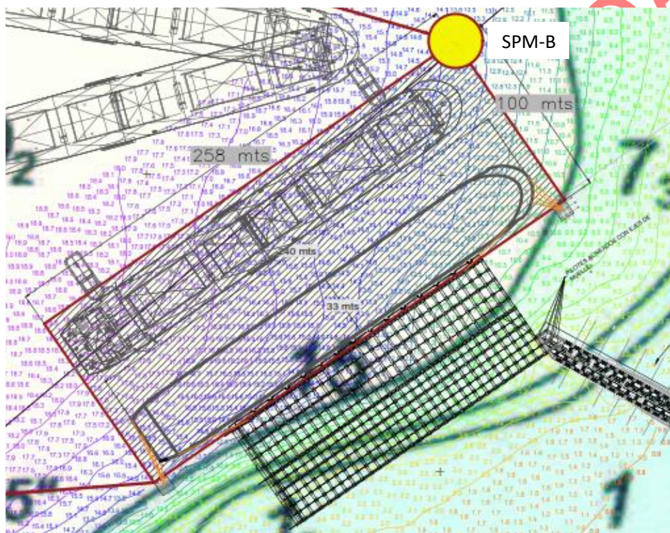
Ilustración 4. Área de aproximación y atraque frente al muelle marítimo de Mardique Fuente: Estudio de Maniobrabilidad Mardique
