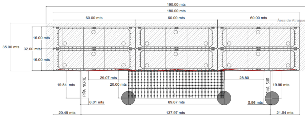
Ilustración 14. Esquema de amarre de un convoy de 4 barcasas Fuente: Estudio de Maniobrabilidad de Mardique
