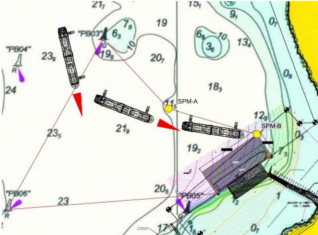
Ilustración 3. Dársena de Maniobras de la Sociedad Portuaria Mardique Fuente: Estudio de Maniobrabilidad Mardique
